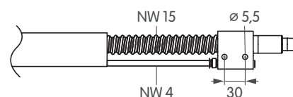
Saug-Blas-Einheit für fixierte Montage
