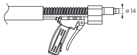
Saug-Blas-Einheit für fixierte Montage
